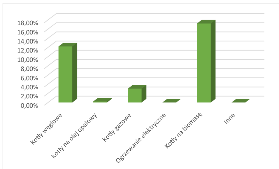
Rysunek 5 Struktura źródeł ciepła w budynkach niedocieplonych
